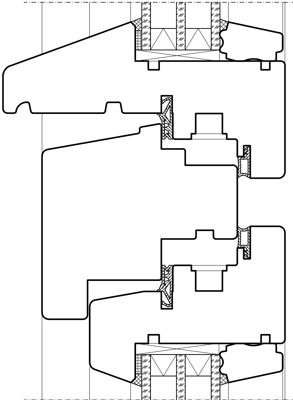
Schnitt Kämpfer
