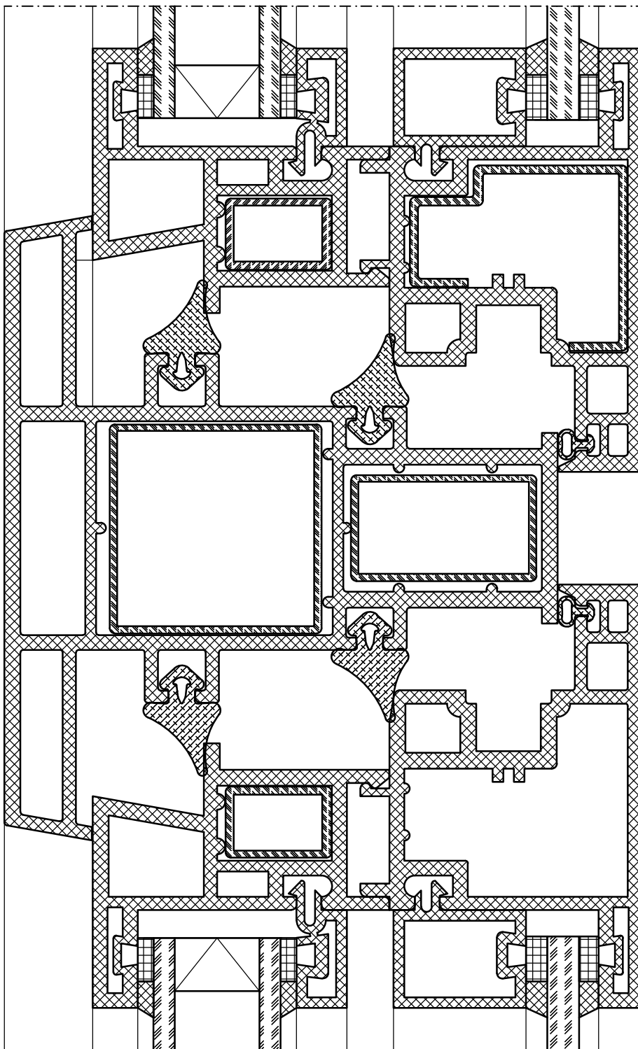
Schnitt Kämpfer
